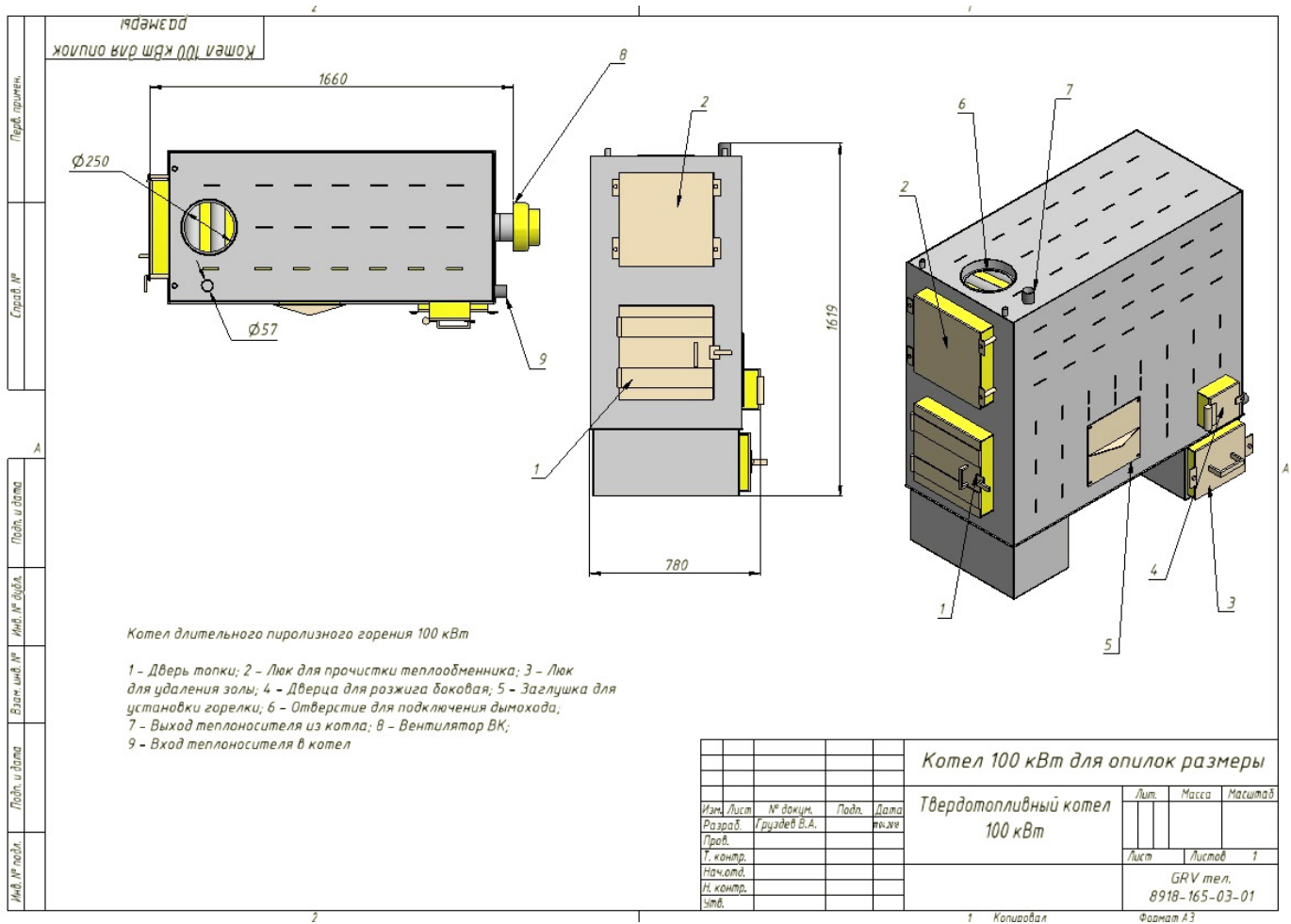
Рис. 3 Габаритные размеры котла универсального 100 кВт
